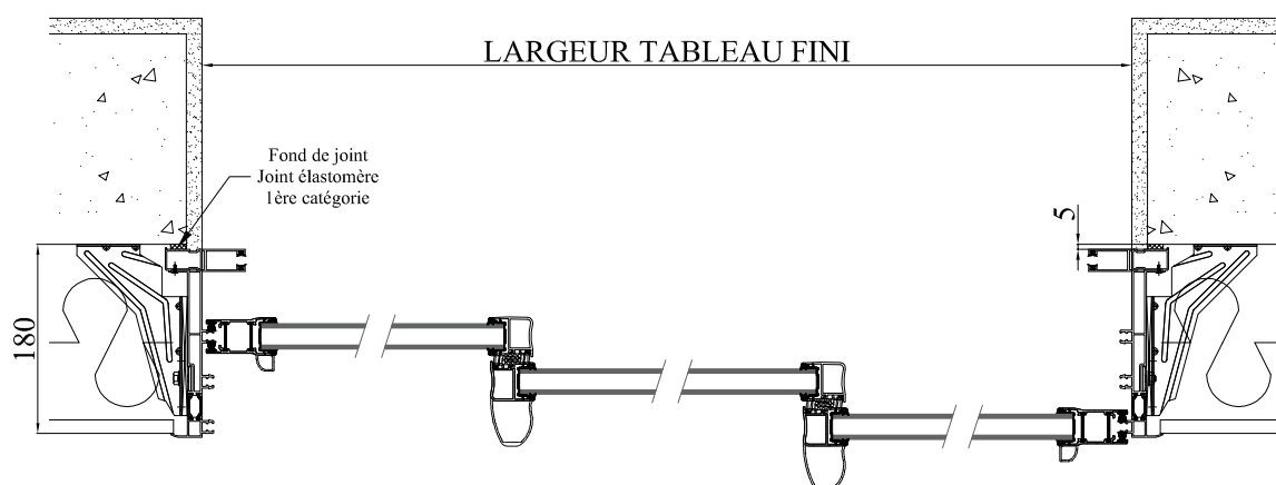
COUPE HORIZONTALE
