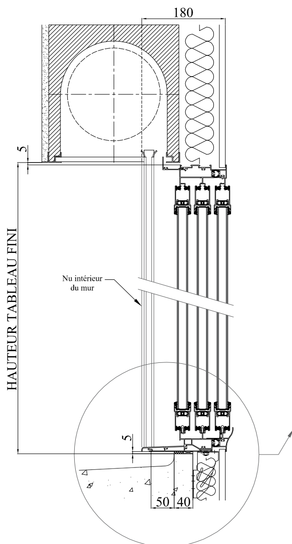
COUPE VERTICALE
