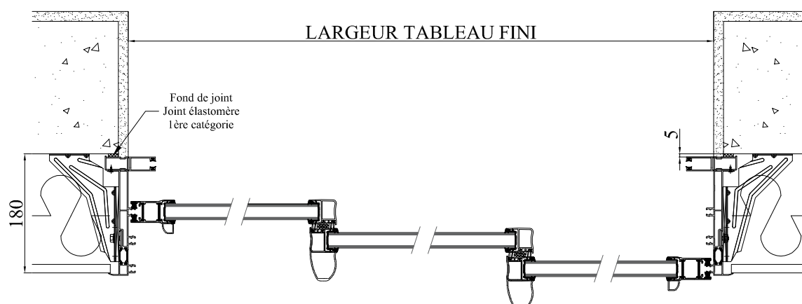
COUPE HORIZONTALE
