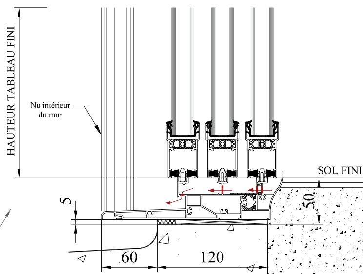
DETAIL PIECE D'APPUI Sans Echelle
