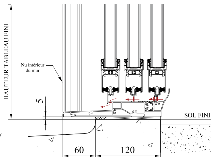
DETAIL PIECE D'APPUI
