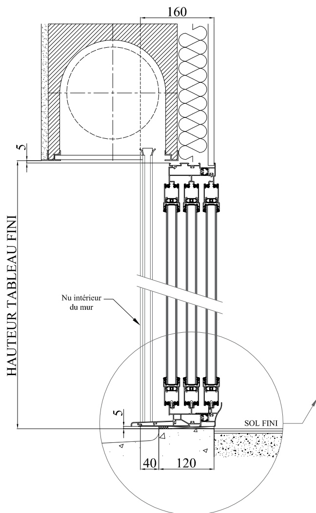
COUPE VERTICALE
