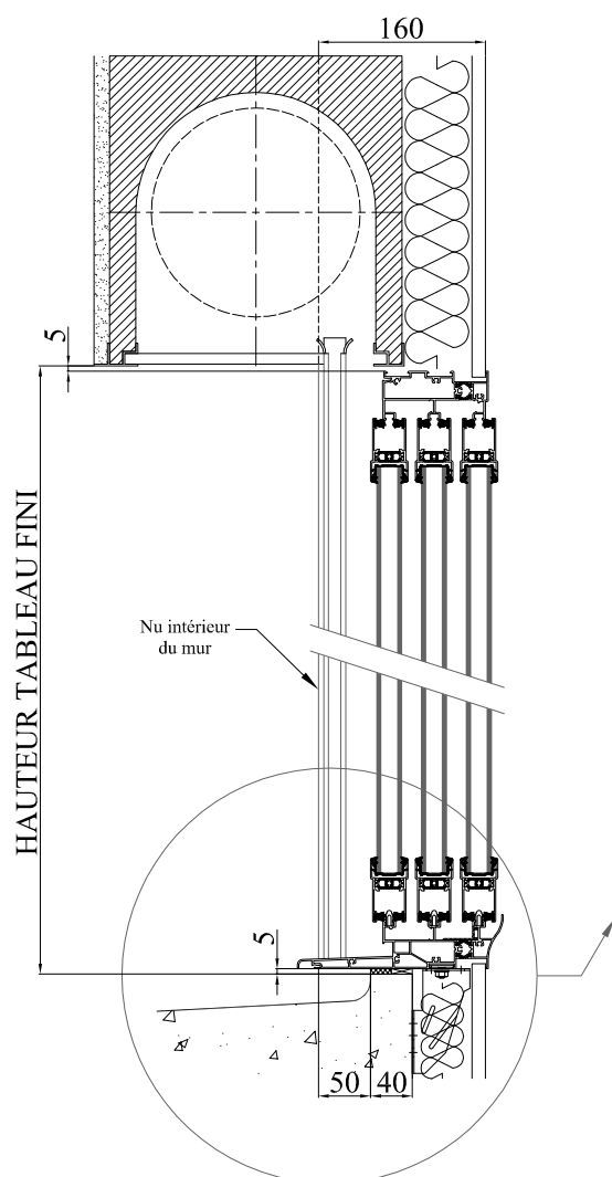
COUPE VERTICALE
