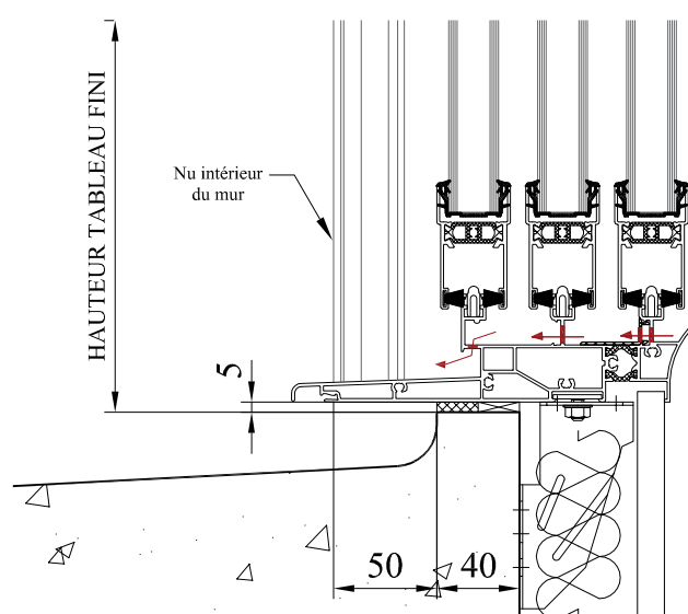
DETAIL PIECE D'APPUI
