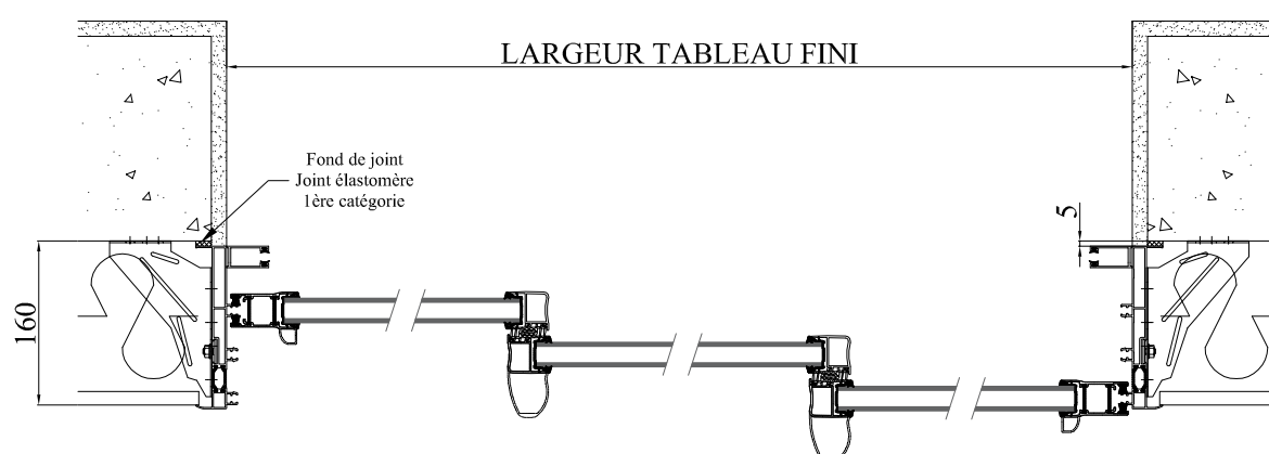
COUPE HORIZONTALE
