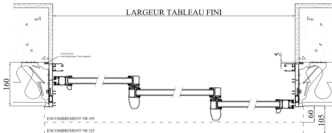
COUPE HORIZONTALE
