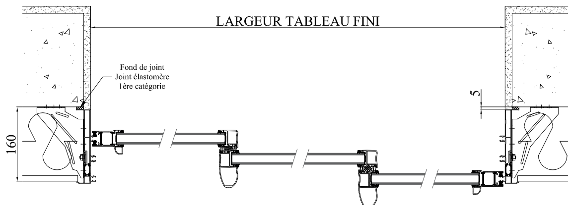
COUPE HORIZONTALE
