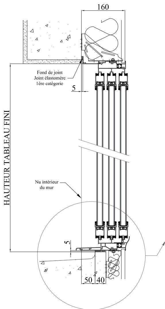
COUPE VERTICALE
