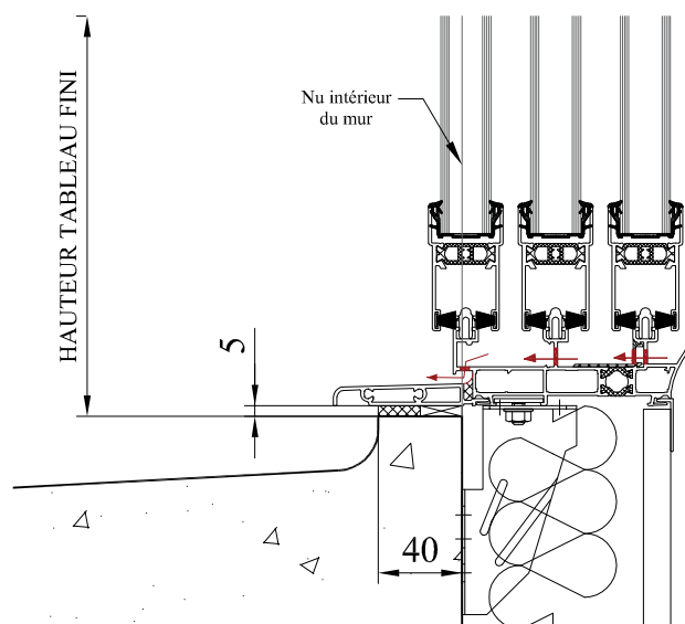
DETAIL PIECE D'APPUI
