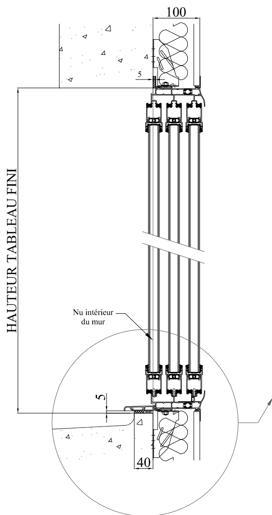
COUPE VERTICALE
