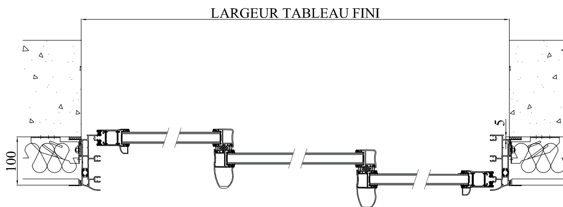
COUPE HORIZONTALE
