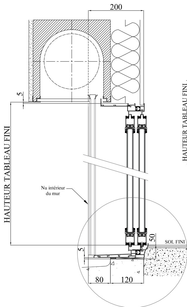
COUPE VERTICALE
