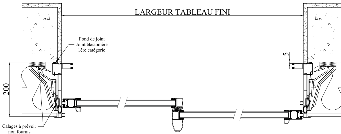
COUPE HORIZONTALE
