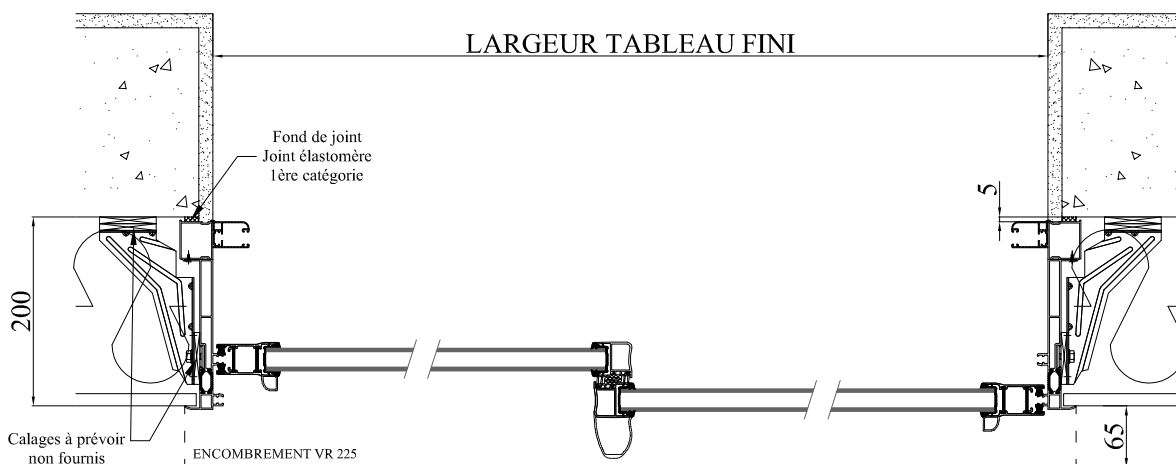
COUPE HORIZONTALE
