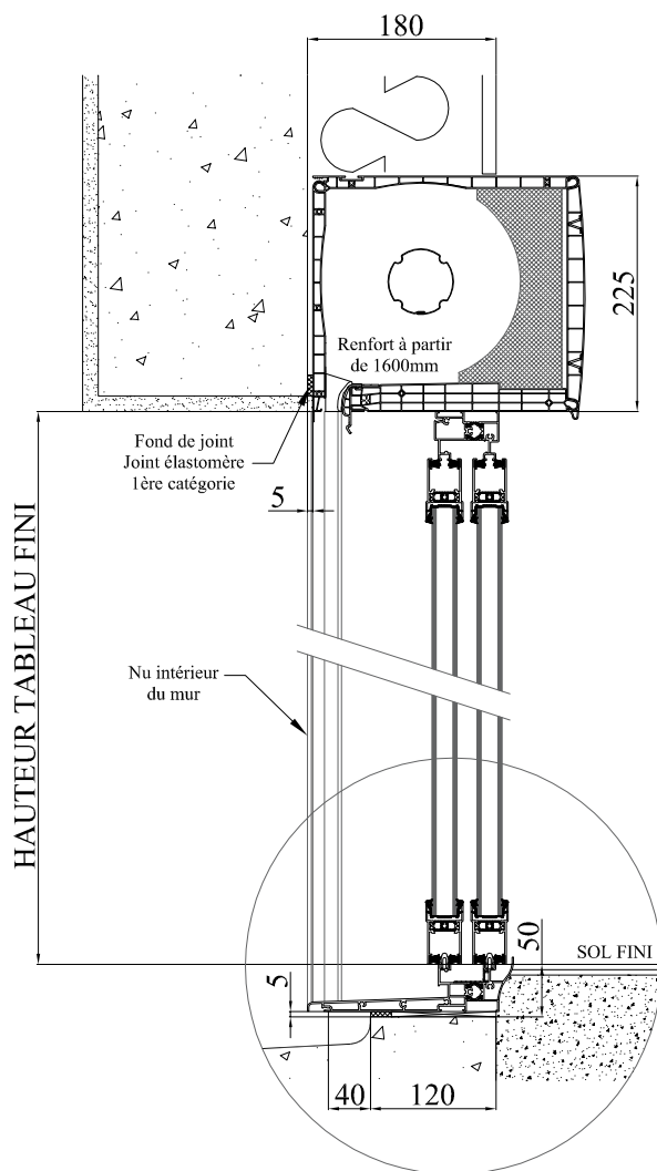
COUPE VERTICALE
