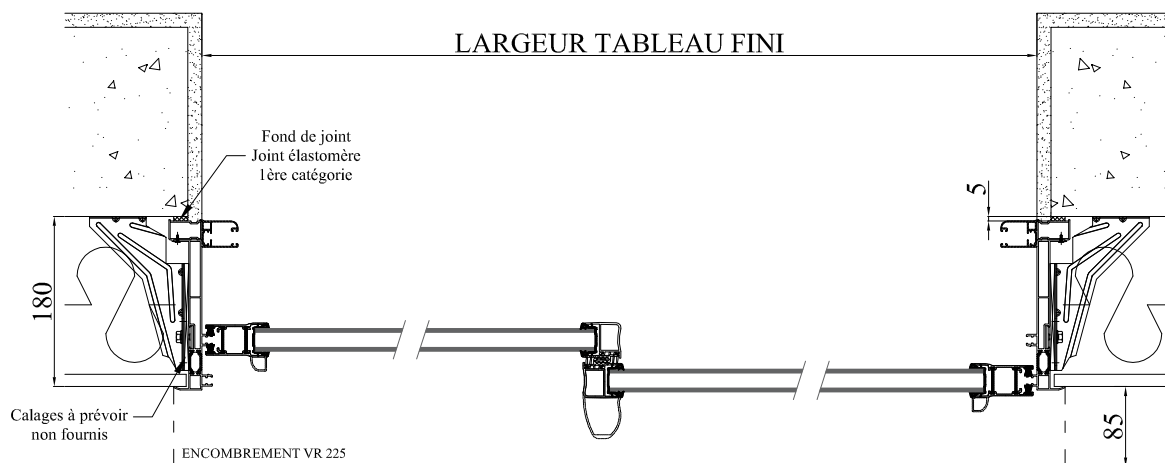
COUPE HORIZONTALE
