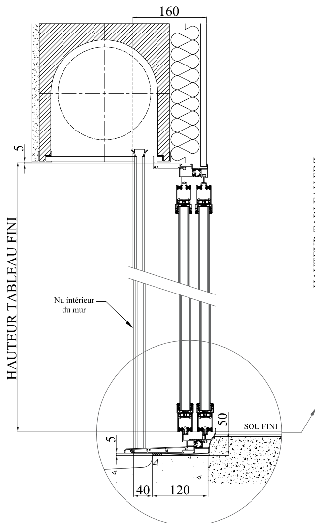
COUPE VERTICALE
