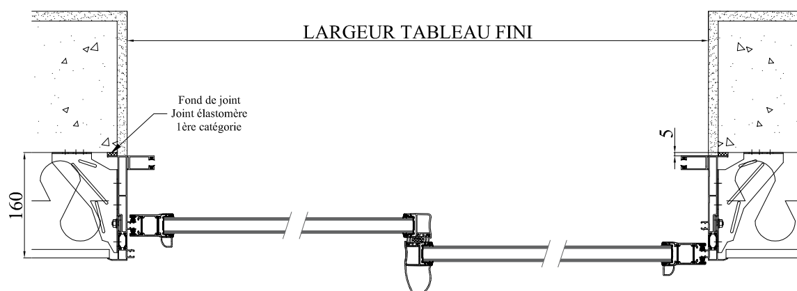
COUPE HORIZONTALE
