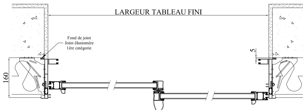
COUPE HORIZONTALE
