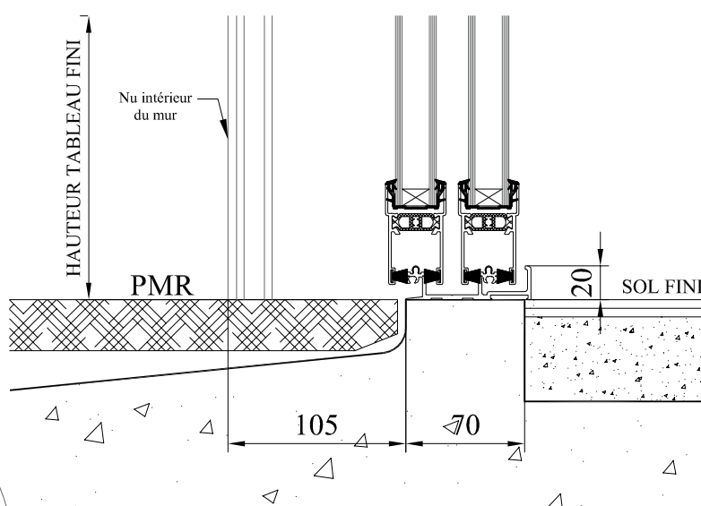
DETAIL PIECE D'APPUI
