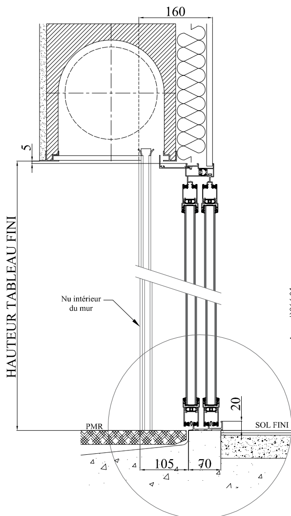
COUPE VERTICALE
