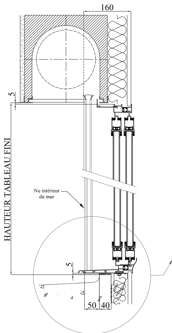
COUPE VERTICALE
