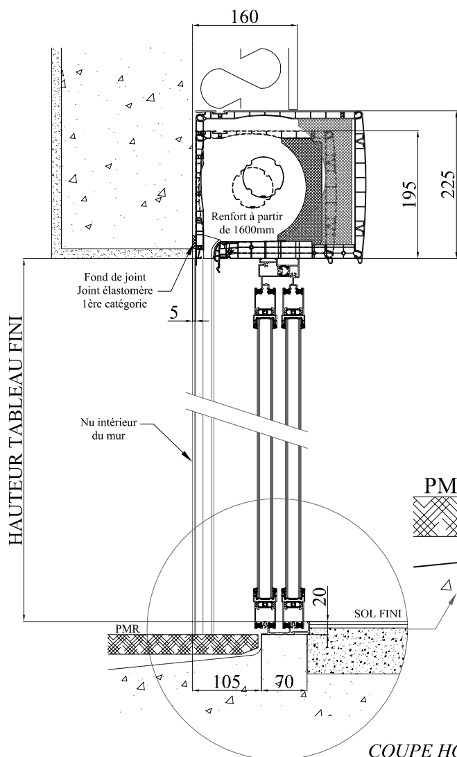
COUPE VERTICALE
