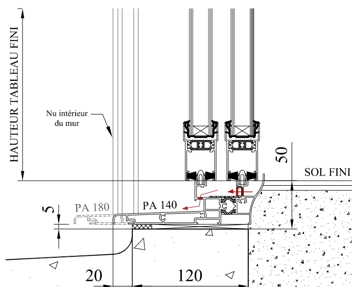
DETAIL PIECE D'APPUI
