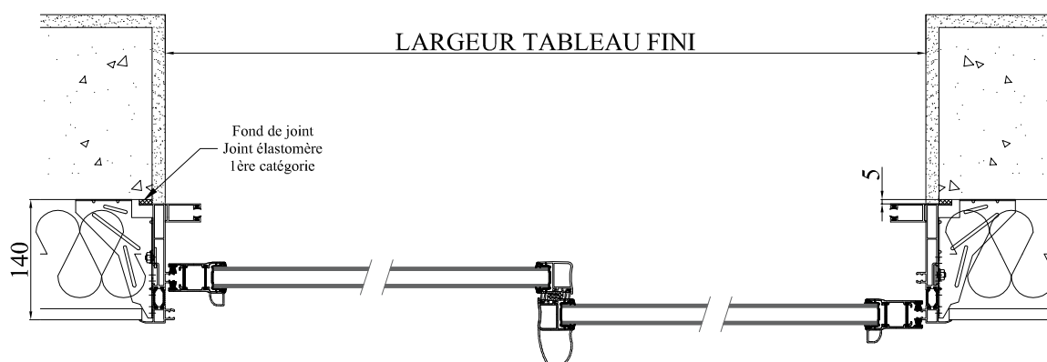
COUPE HORIZONTALE
