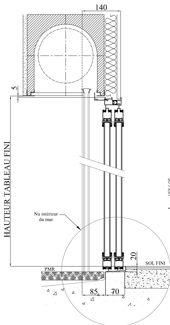
COUPE VERTICALE
