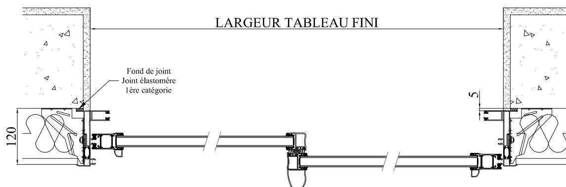
COUPE HORIZONTALE
