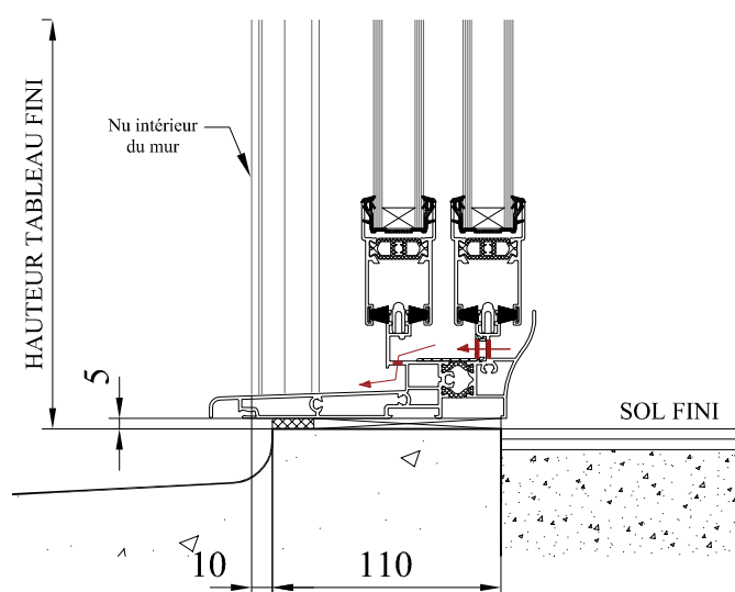
DETAIL PIECE D'APPUI
