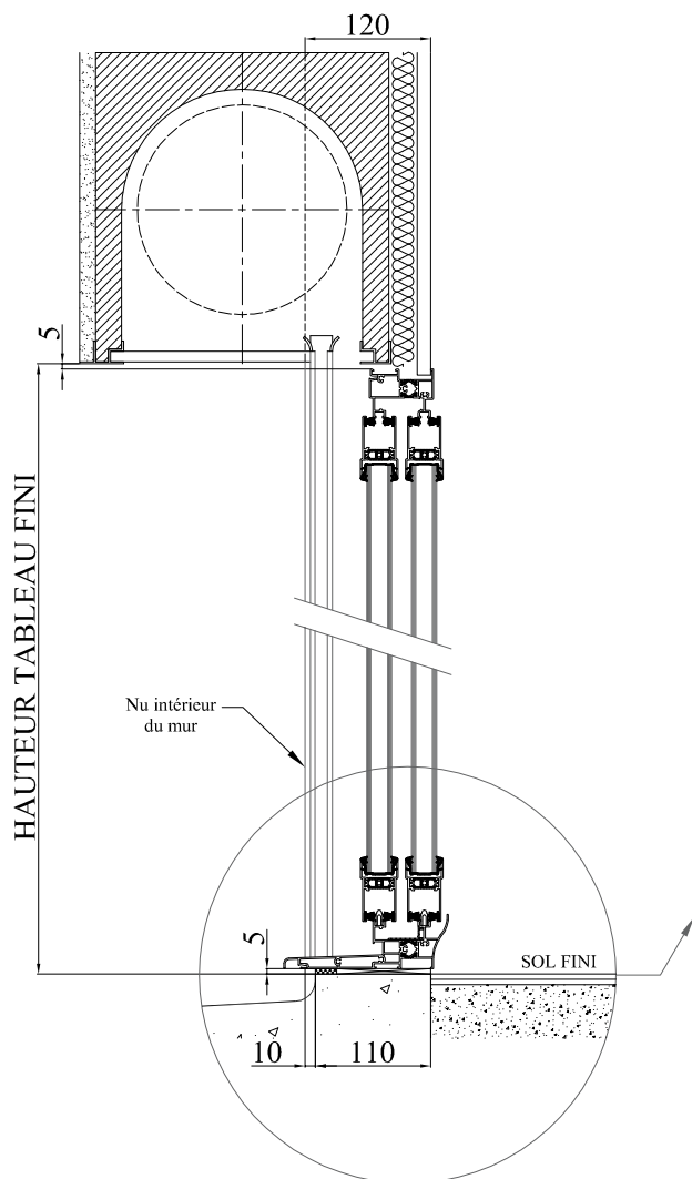
COUPE VERTICALE
