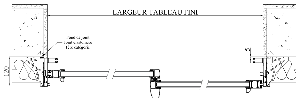
COUPE HORIZONTALE
