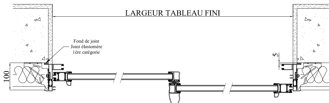
COUPE HORIZONTALE
