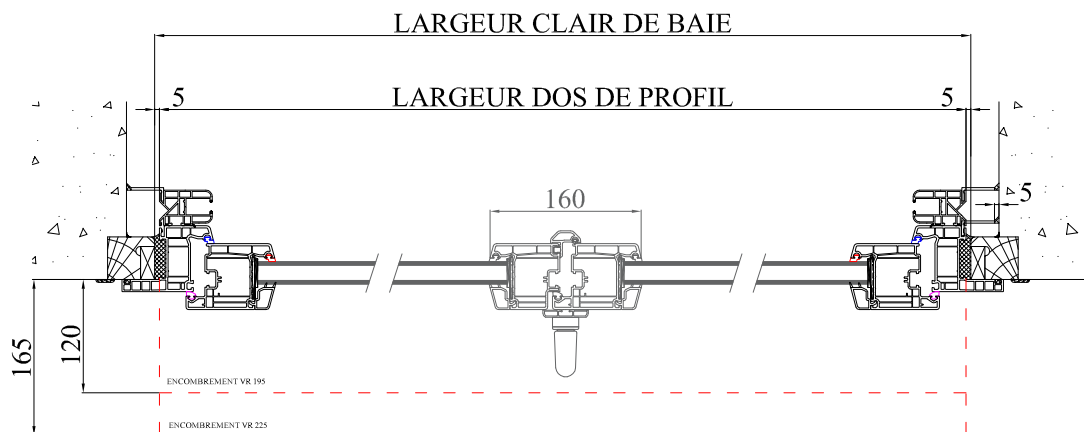
COUPE HORIZONTALE
