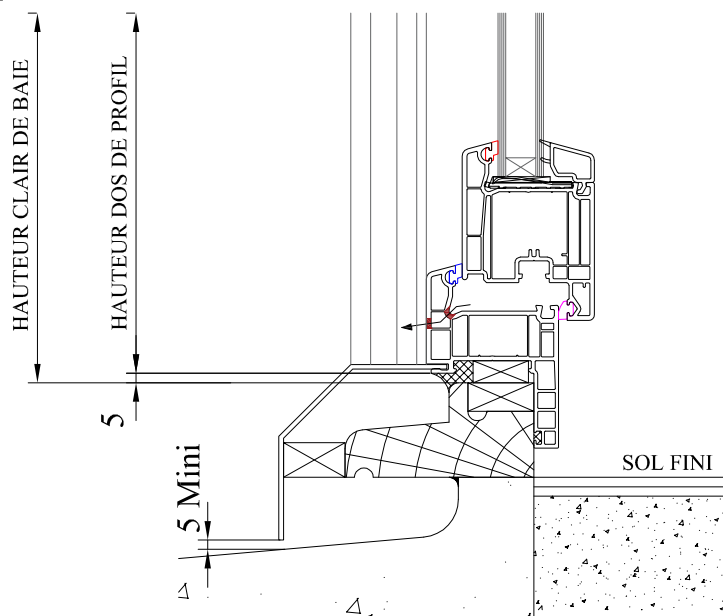
DETAIL PIECE D'APPUI
