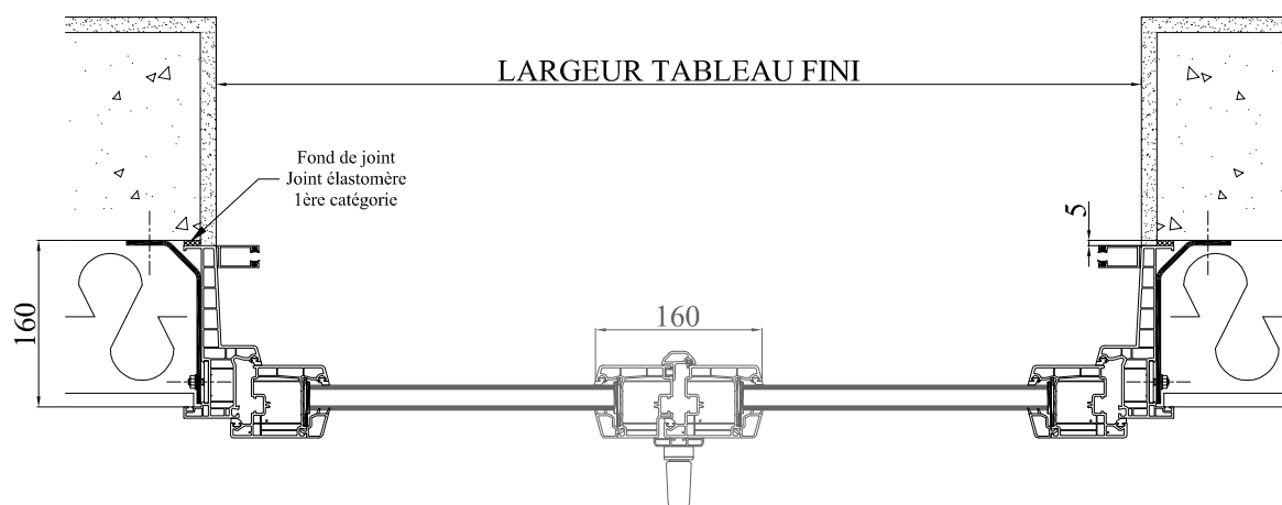
COUPE HORIZONTALE
