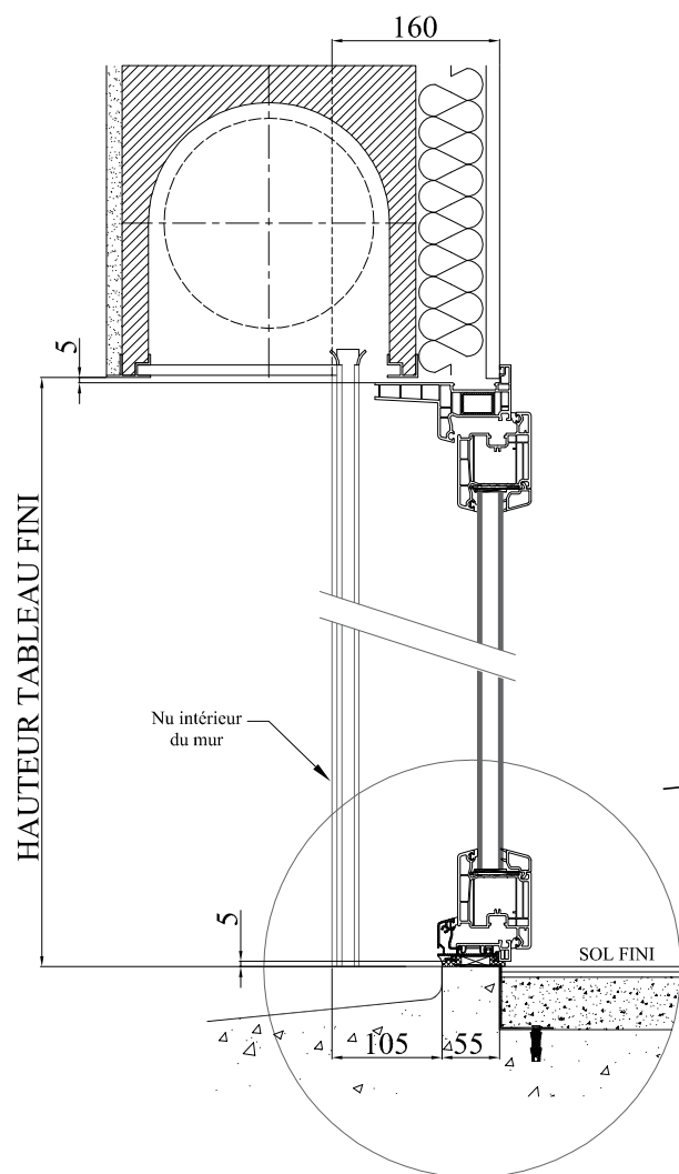
COUPE VERTICALE
