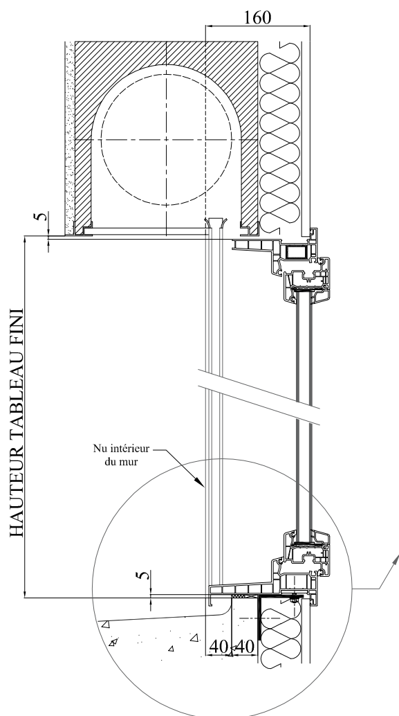
COUPE VERTICALE
