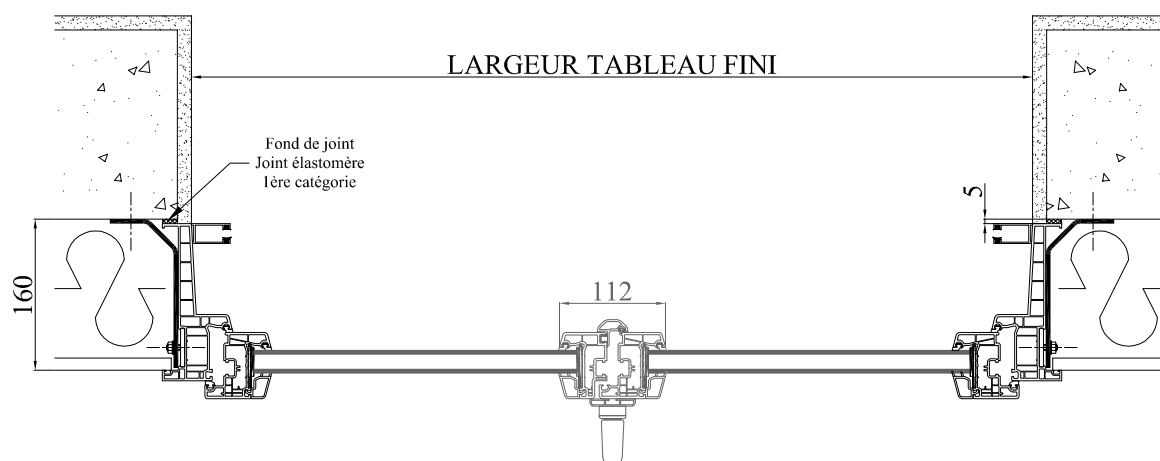
COUPE HORIZONTALE
